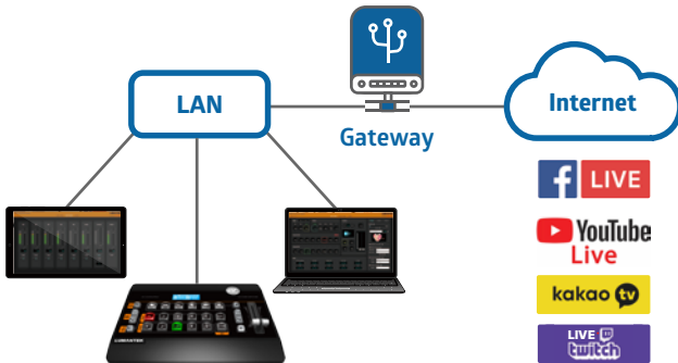
[그림 1-1] VS5 네트워크 구성 예
